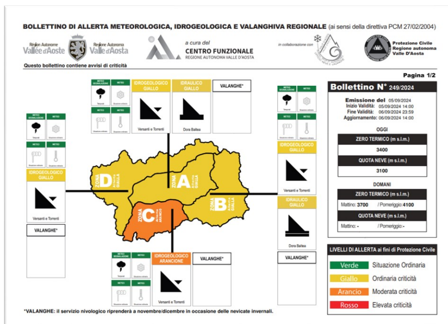
Fig. 1 – Estratto del bollettino di allertamento del 5 settembre 2024
